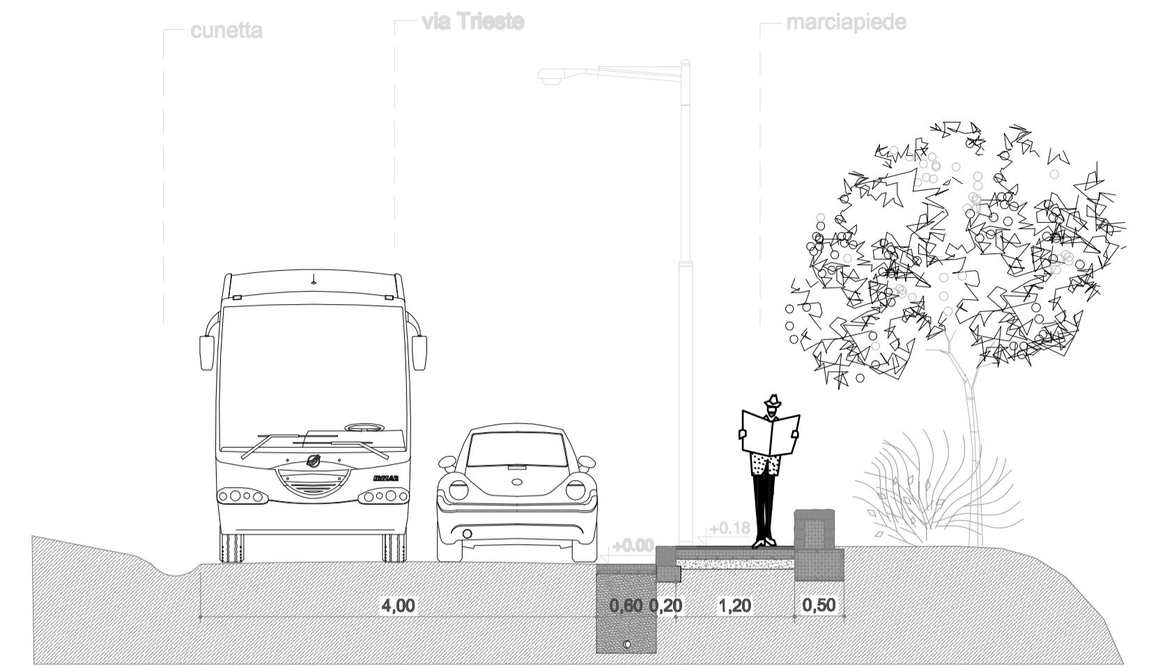
SEZIONE TRASVERSALE A-A scala 1:50
