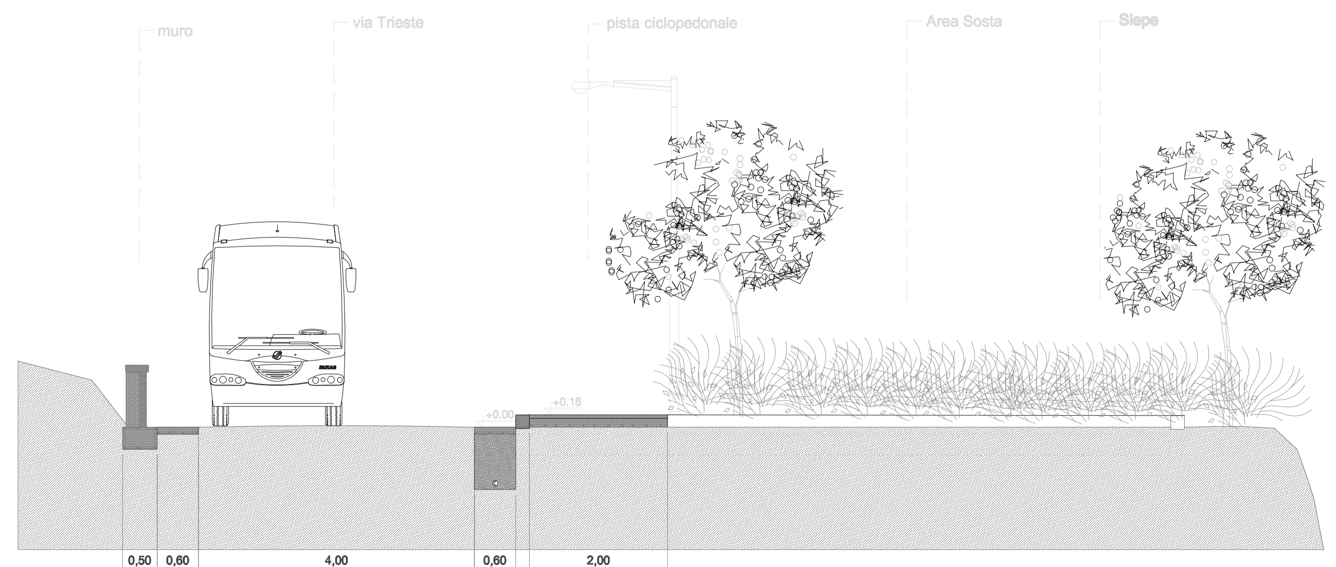
SEZIONE TRASVERSALE B-B scala 1:50
